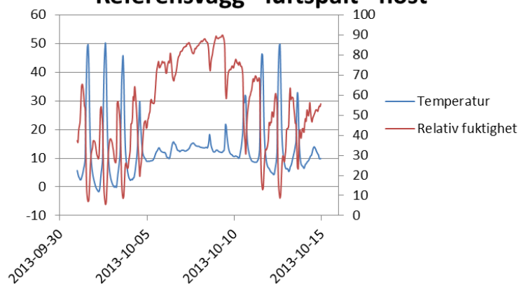
Figur 12. Temperatur och relativ fuktighet i luftspalt bakom träpanel hos referensvägg. Figuren visar två veckor under hösten 2013.
