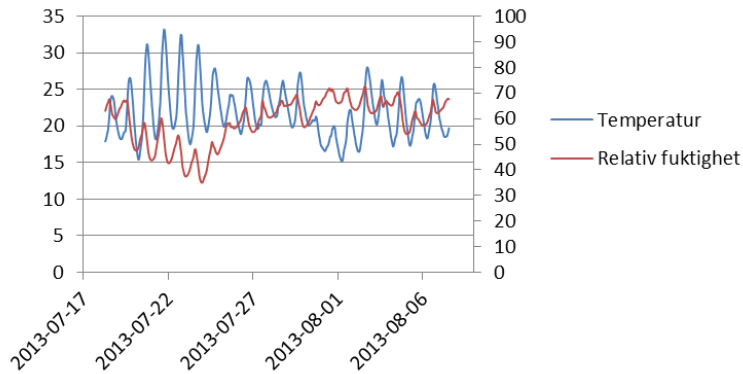
Figur 11. Temperatur och relativ fuktighet i mineralull bakom vindskiva (motsvarande position för yttre läkt) hos grön vägg. Figuren visar två veckor under sommaren 2013.
