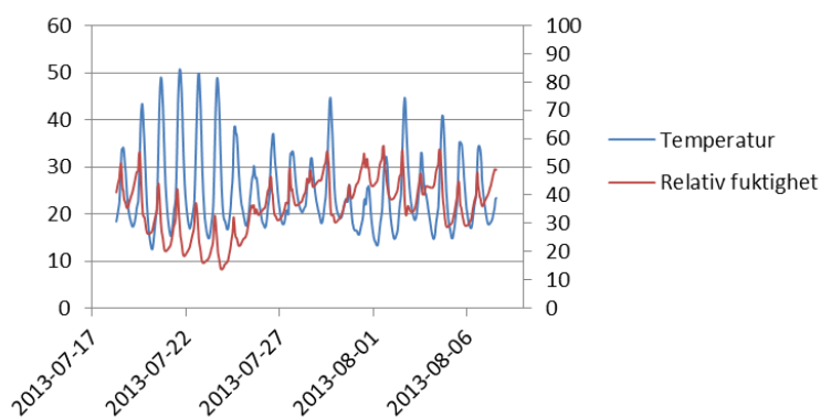
Figur 10. Temperatur och relativ fuktighet i mineralull bakom vindskiva hos referensvägg (motsvarande position för yttre läkt). Figuren visar två veckor under sommaren 2013.
