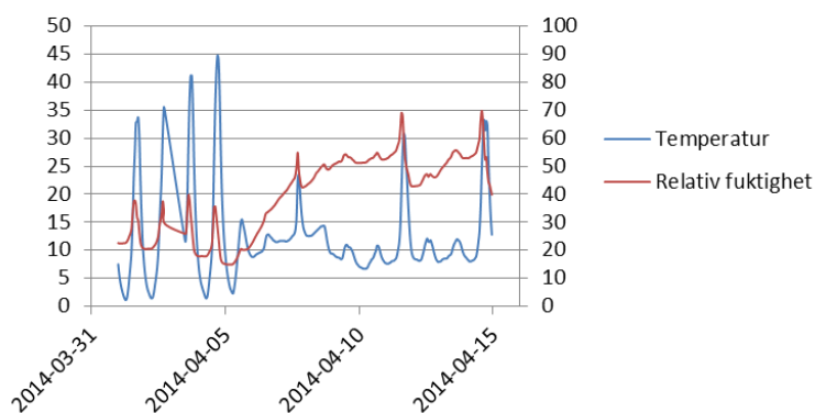
Figur 22. Temperatur och relativ fuktighet i mineralull bakom vindskiva hos referensvägg (motsvarande position för yttre läkt). Figuren visar två veckor under våren 2014.
